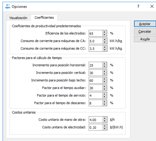
Figura 10 Cuadro de diálogo de especificación de coeficientes
