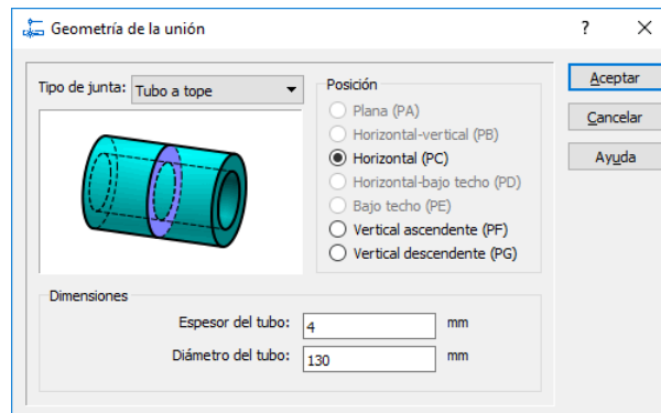
Figura 4 Diálogo para la entrada de datos de la geometría de la unión
